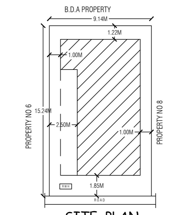
SITE PLAN 1:200
